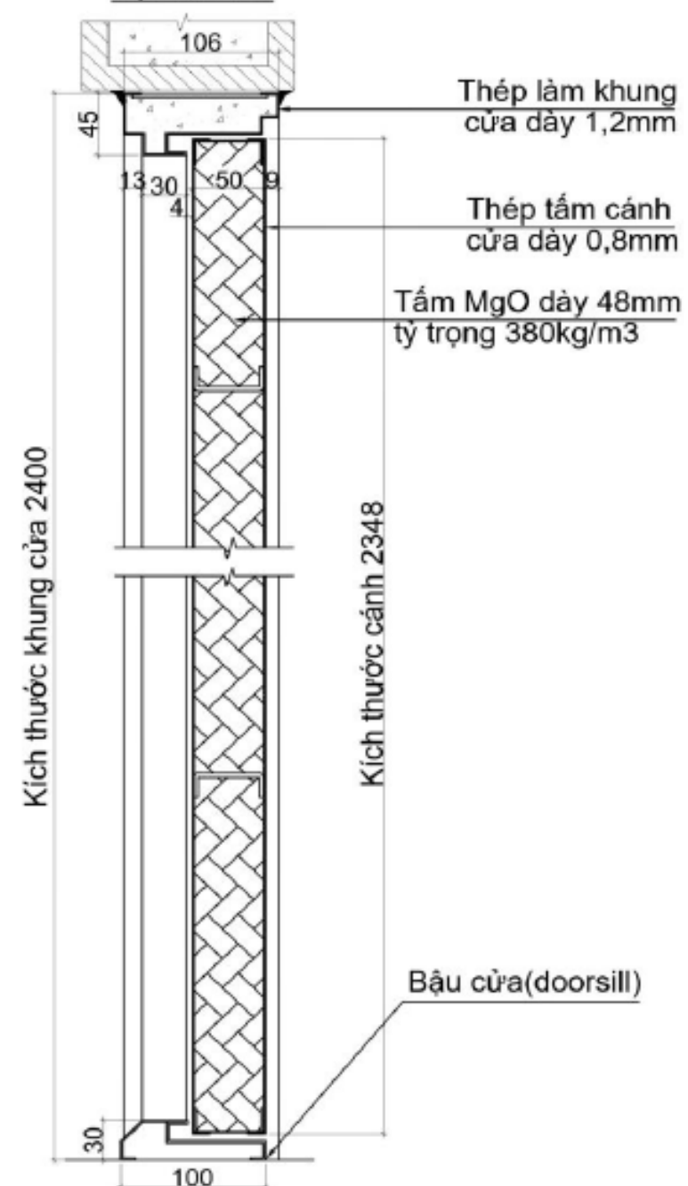
MẶT CẮT B-B
