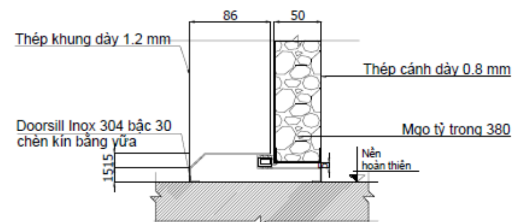
CHI TIẾT II
