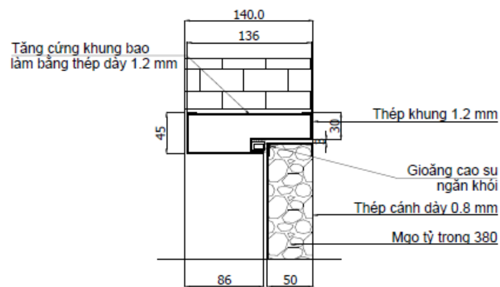
CHI TIẾT I
