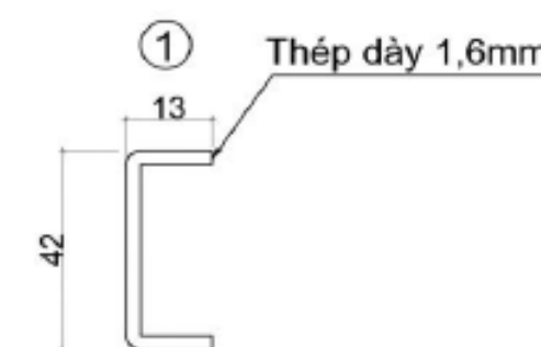
XUỐNG TĂNG CỨNG TÂM CẢNH CỬA
