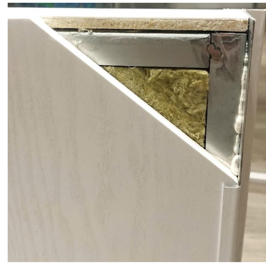
4. Kết cấu Cánh HGF Laminate
