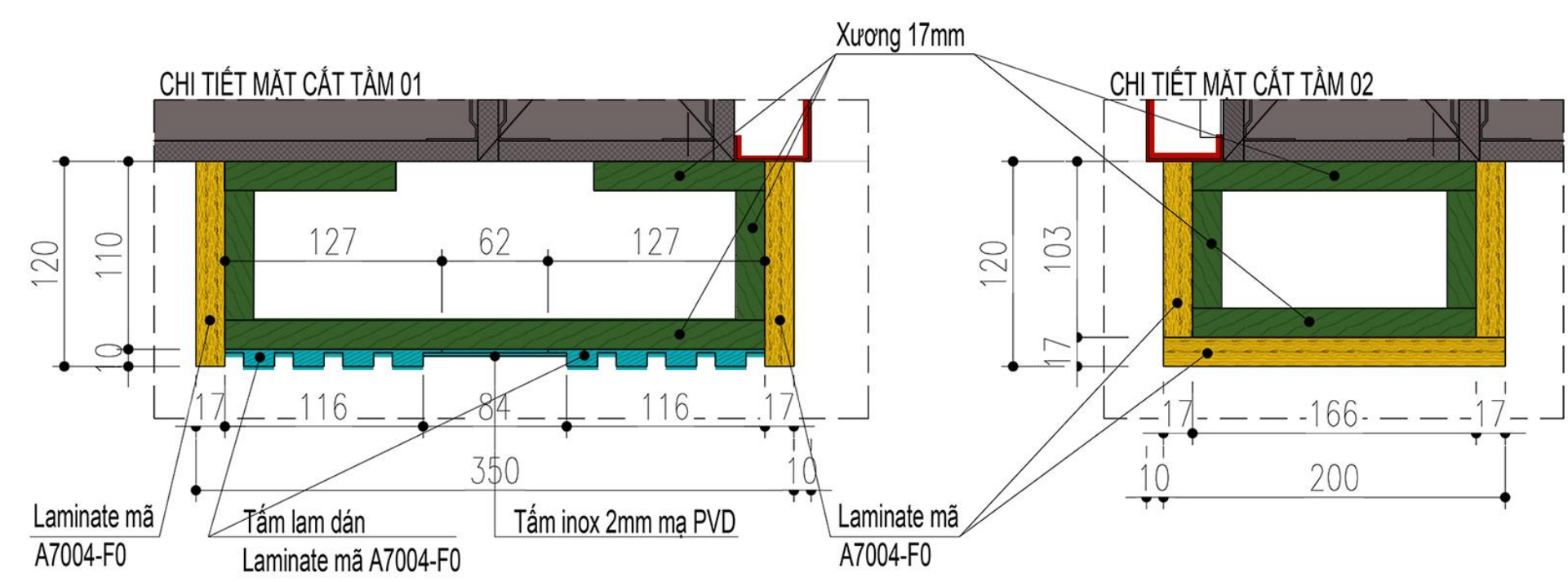
MẶT CẮT B
