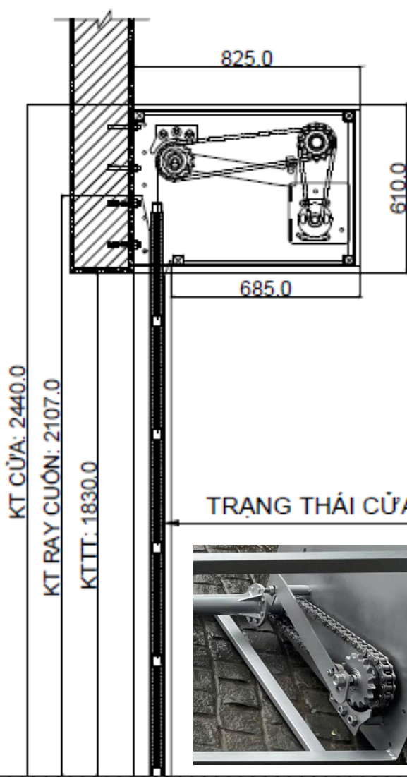
MẶT CẮT B-B
